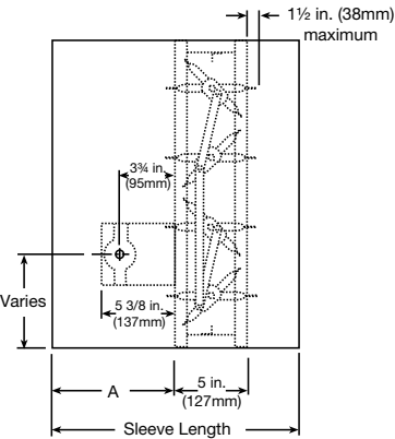
Sideplate
