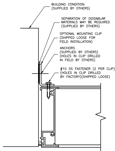
JAMB DETAIL
