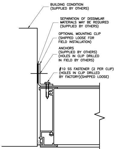
JAMB DETAIL
